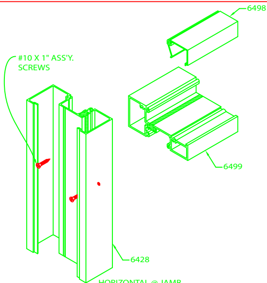
HORIZONTAL @ JAMB
