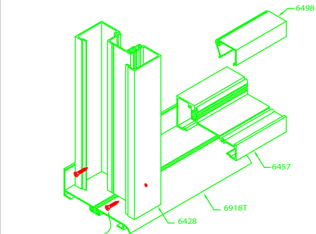
SILL @ JAMB
